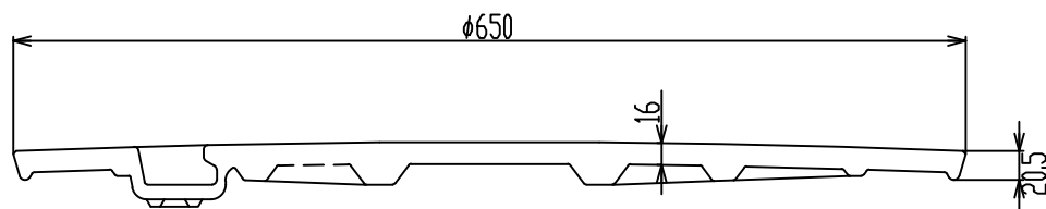
A-A' 断面
