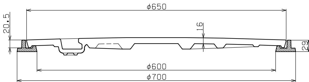
A-A' 断面図
