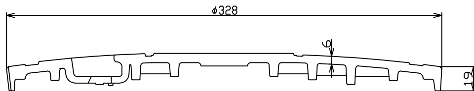
A-A' 断面図
