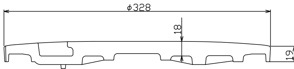
A - A' 断面
