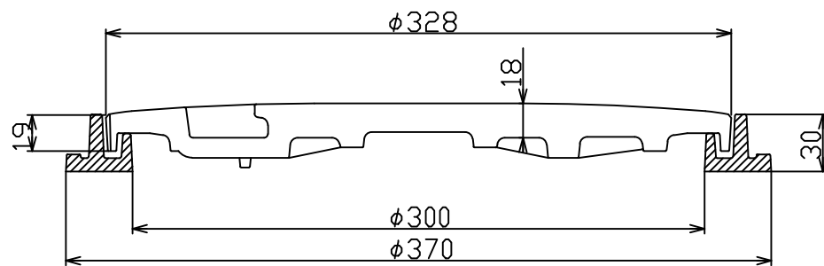
A - A' 断面図
