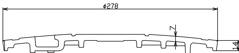
A-A' 断面図
