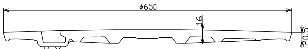
A-A' 断面
