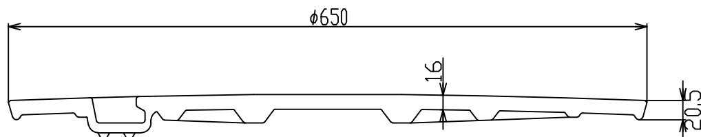
A-A' 断面
