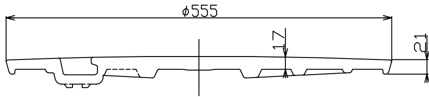
A-A' 断面図
