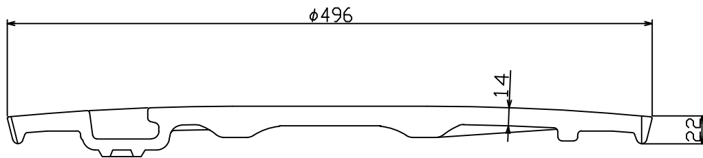
A-A' 断面図
