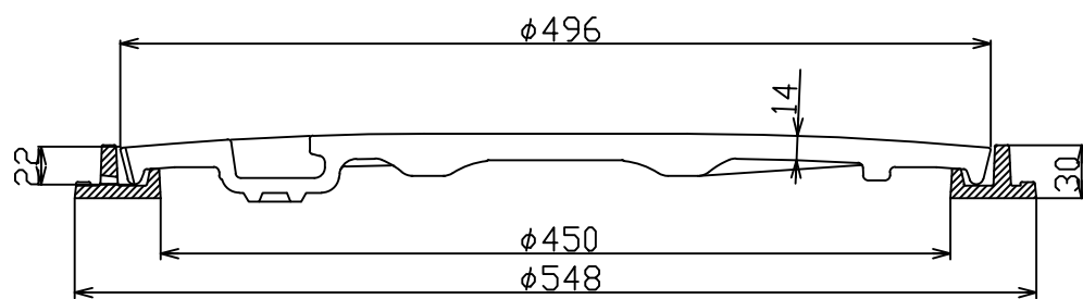
A-A' 断面図
