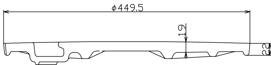
A-A' 断面図
