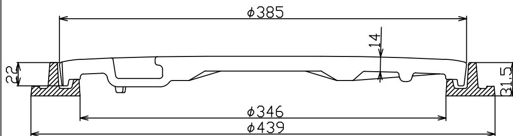
A-A' 断面図
