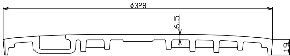
A-A' 断面図
