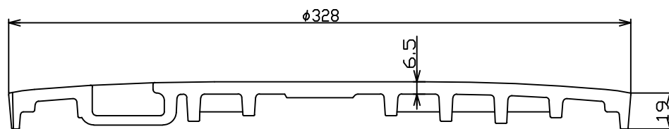
A-A' 断面图
