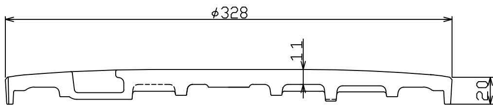
A-A' 断面図
