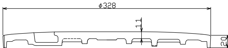
A-A' 断面図
