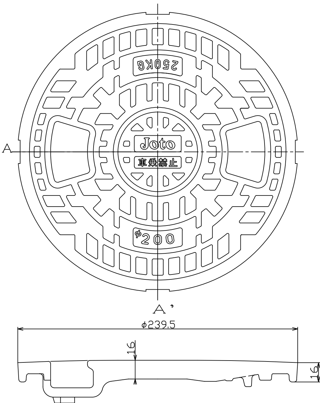
A - A' 断面
