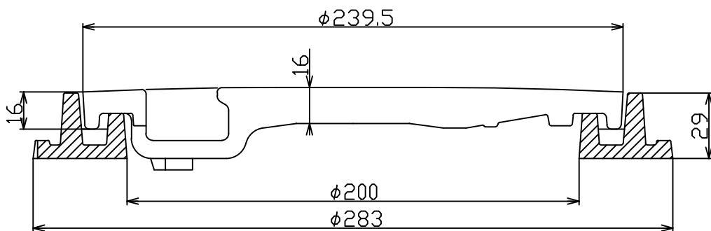
A - A' 断面
